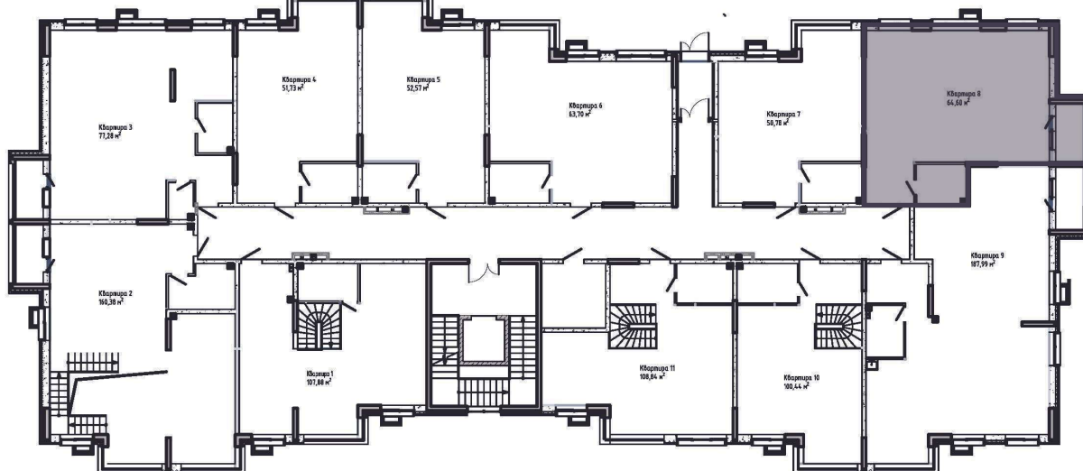
План 1-го этажа, МКД 1,3
