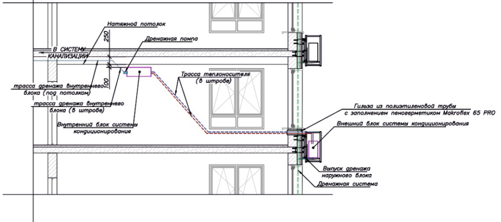
Вариант 3. Выпуск внутреннего дренажа с помпой в систему канализации
